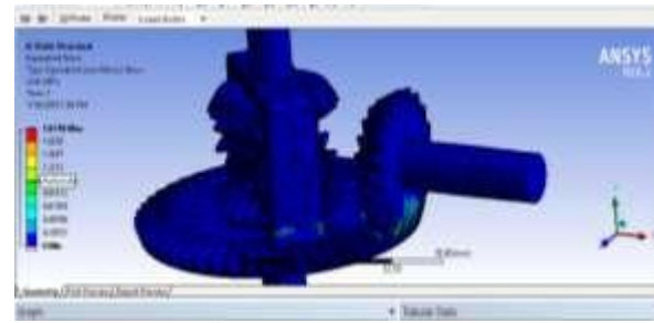
fig 2.7 von mises stress
